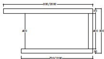
Vista frontale
